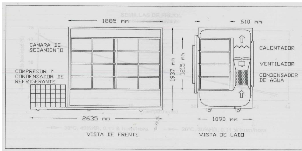
Figura 14. Diagrama del secador de aire fresco (SAF).
